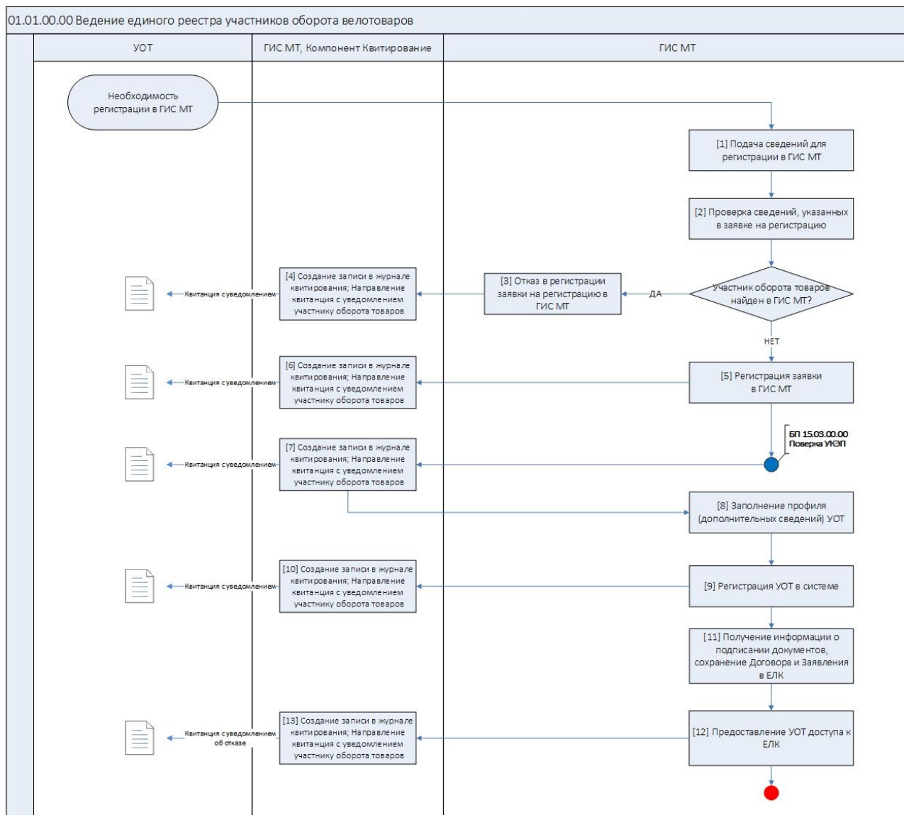
Рисунок 1 Схема процесса 01.01.00.00 Ведение единого реестра участников оборота велотоваров.
