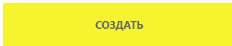
Рисунок 6. Кнопка «Создать»
