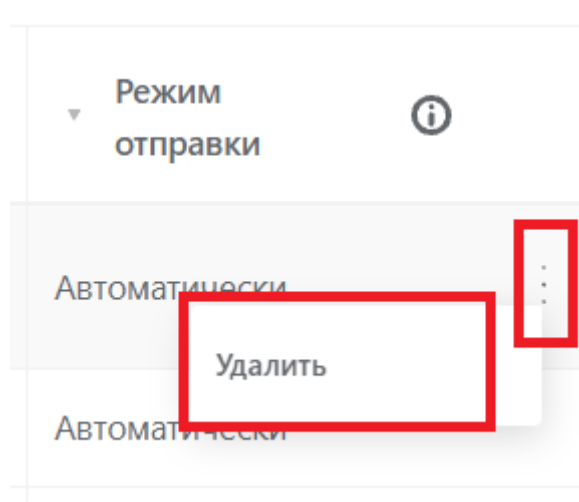
Рисунок 7. Кнопка «Удалить»
