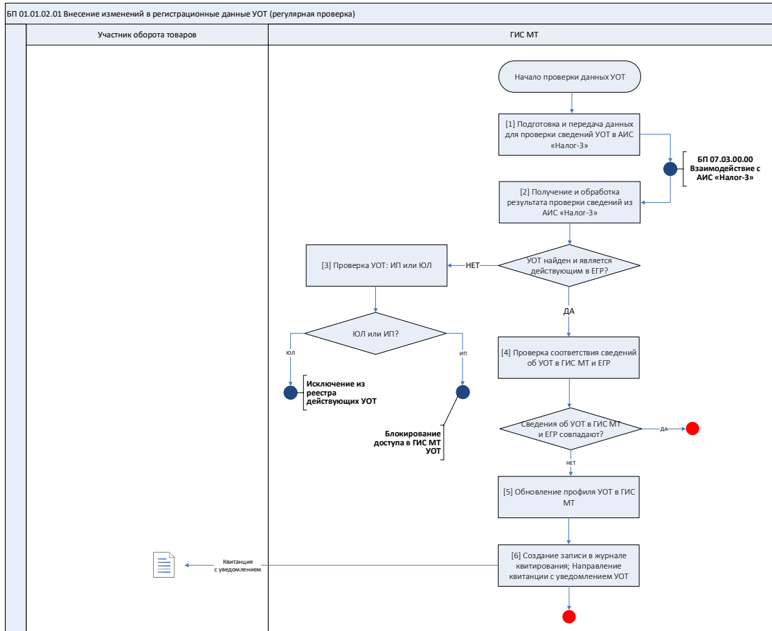
Рисунок 2 Схема процесса 01.01.02.01 Внесение изменений в регистрационные данные участника оборота товаров (регулярная проверка)
