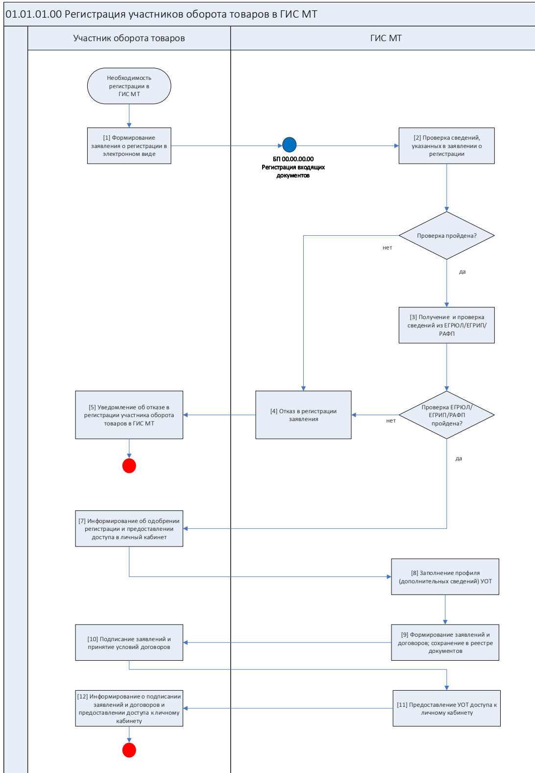
Рисунок 1 Схема процесса 01.01.01.00 Регистрация участников оборота товаров
