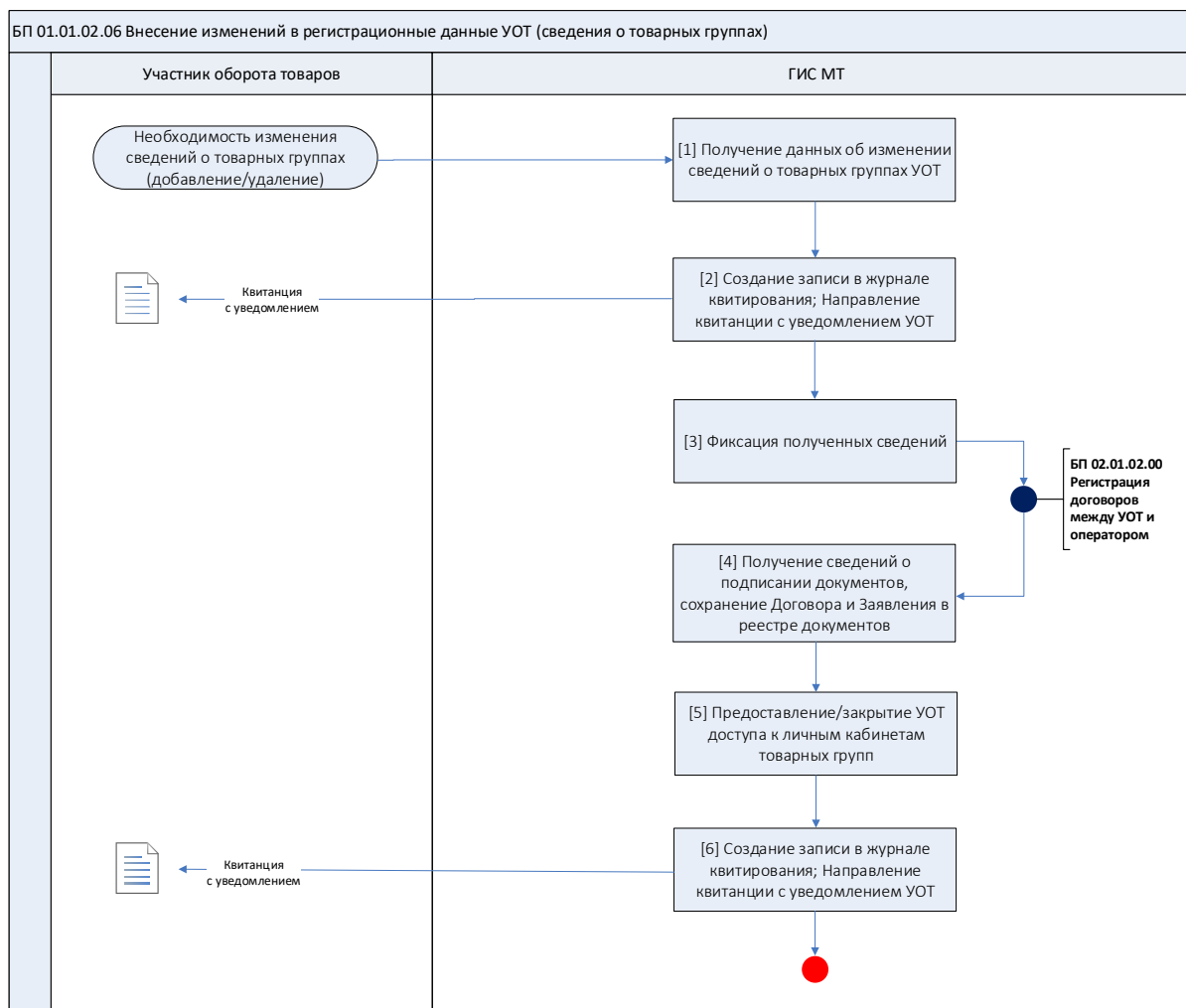
Рисунок 7 Схема процесса 01.01.02.06. Внесение изменений в регистрационные данные участника оборота товаров (товарные группы)
