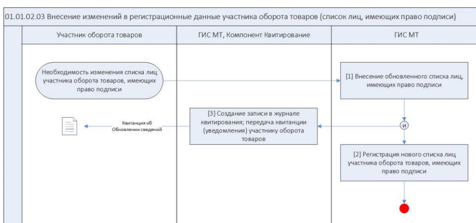
Рисунок 4 Схема процесса 01.01.02.03 Внесение изменений в регистрационные данные участника оборота товаров (список лиц, имеющих право подписи)
