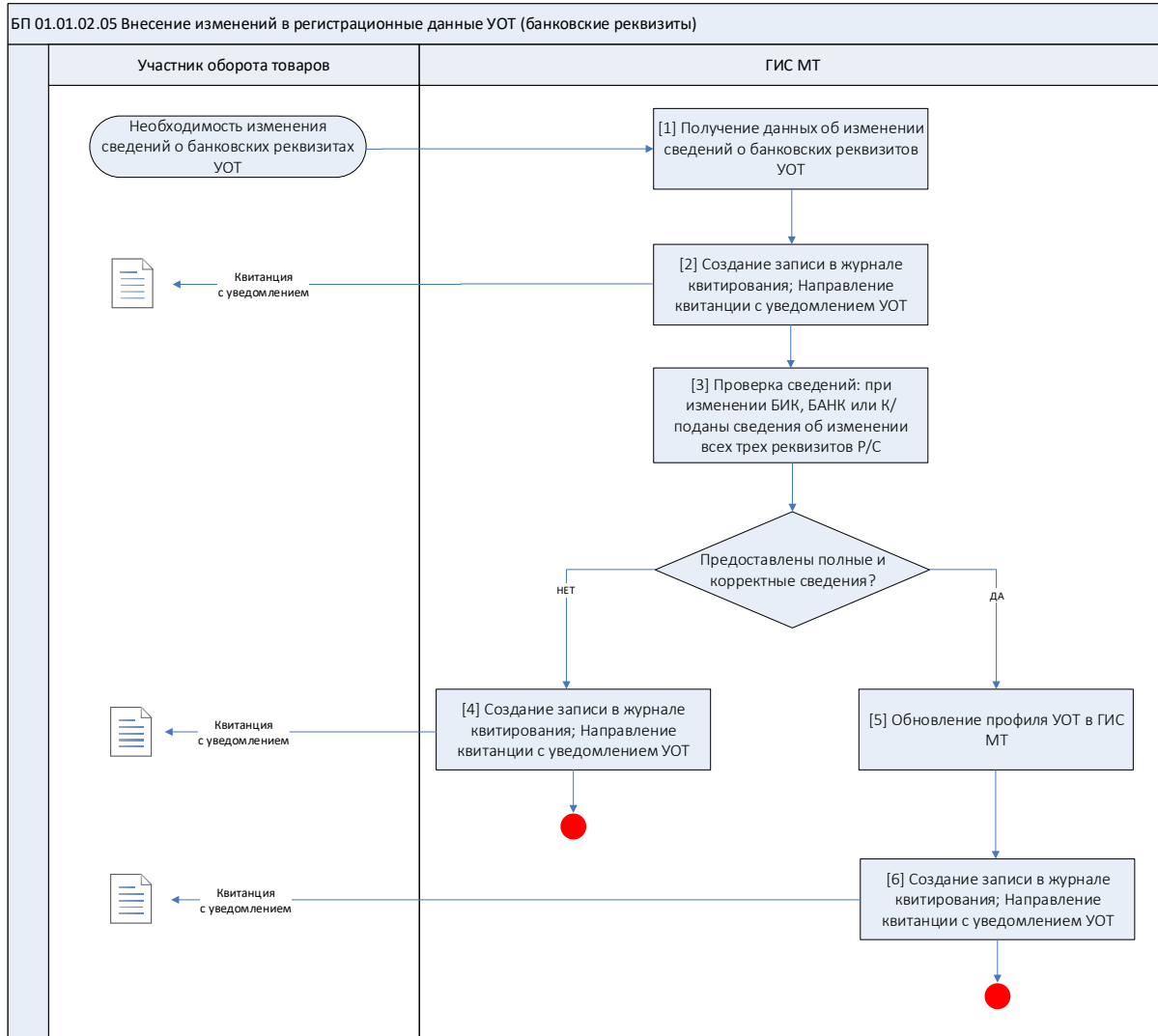
Рисунок 6 Схема процесса 01.01.02.05 Внесение изменений в регистрационные данные участника оборота товаров (банковские реквизиты)
