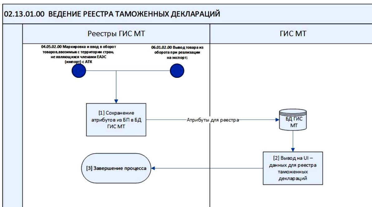
Рисунок 1 Схема процесса
